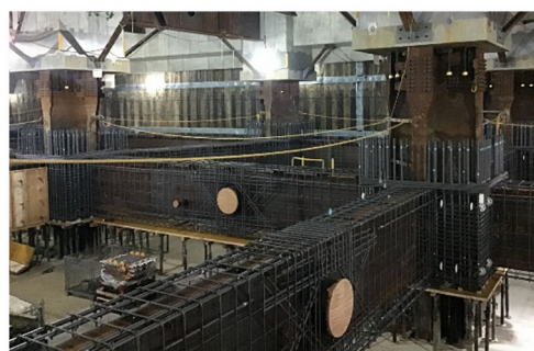
地下1階躯体工事状況
