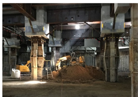
地下1階掘削工事状況
